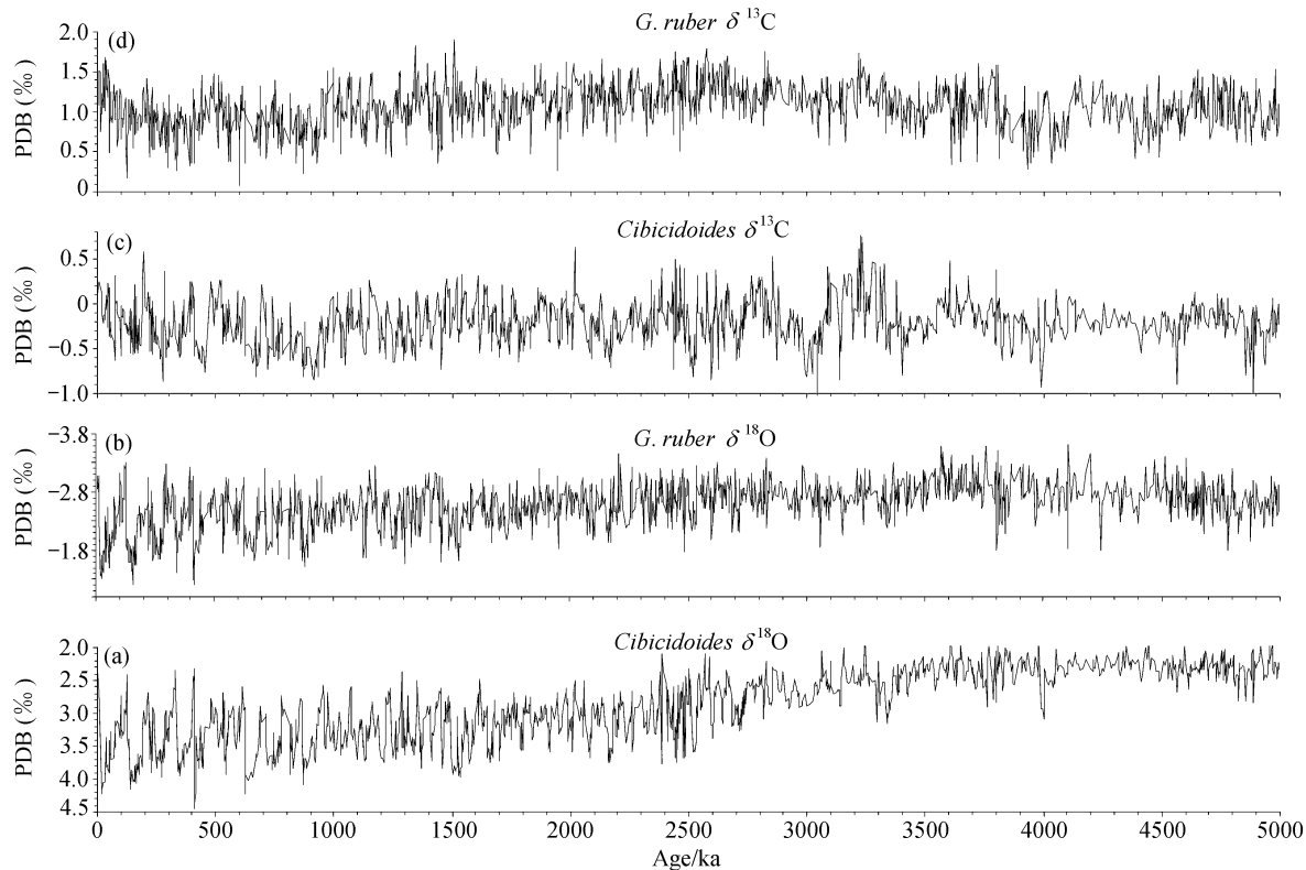
Fig. 1. 5 Ma isotope records from ODP Site 1143. (a) Benthic \delta^{18}\text{O} of Cibicidoides spp.; (b) planktonic \delta^{18}\text{O} of Globigerinoides ruber ; (c) benthic \delta^{13}\text{C} of Cibicidoides spp.; (d) planktonic \delta^{13}\text{C} of Globigerinoides ruber [11,13] .
