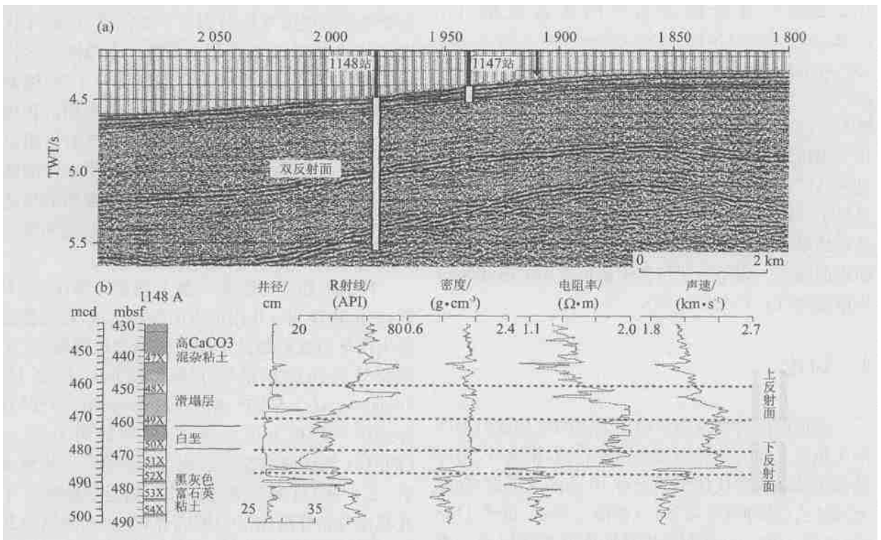
图 4 (a) 地震剖面上的双反射面; (b) 440 ~ 500 mcd 井段的录井曲线 (Wang et al., 2000)
