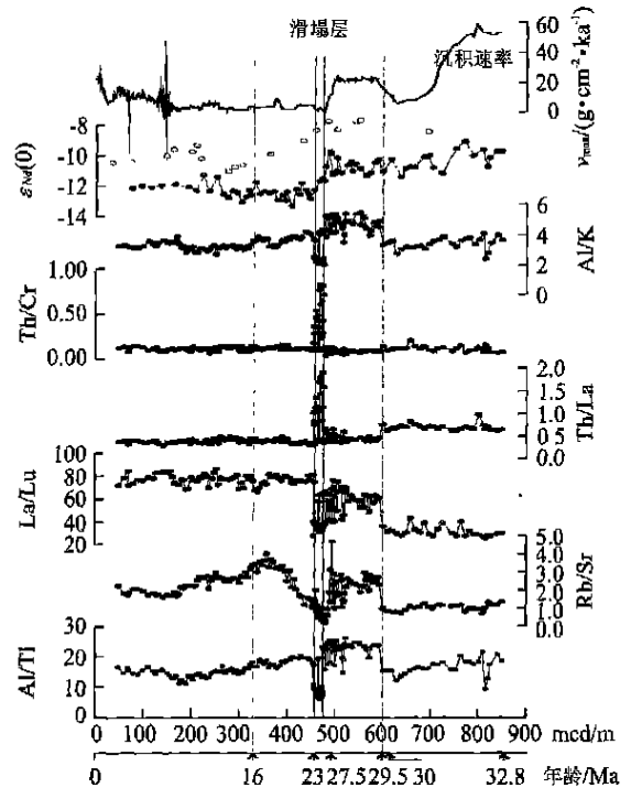
图 5 微量元素比值和 Nd 同位素变化(Li et al. , 2003)
