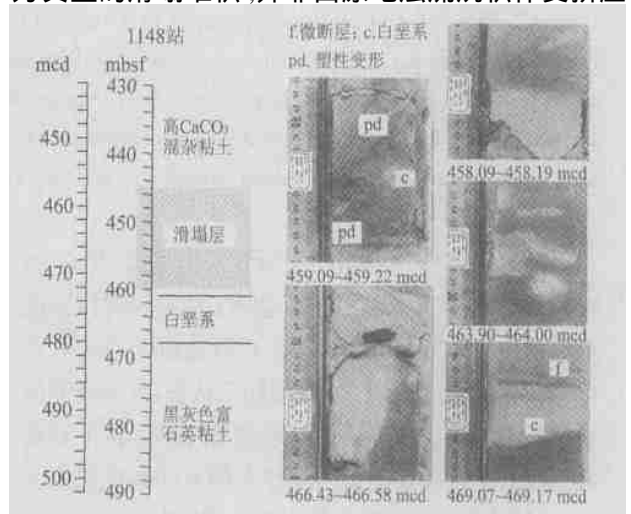
图 2 1148 站滑塌层沉积结构
